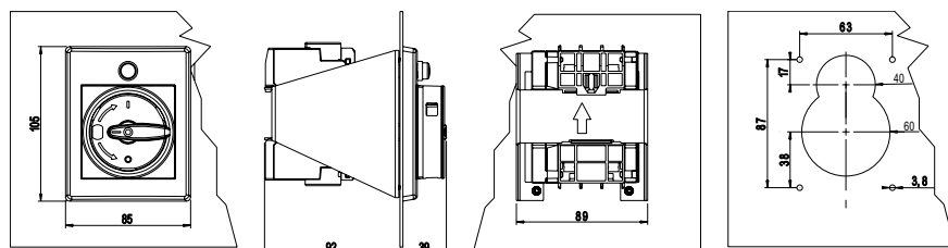
Frontal plate FMEE55E
