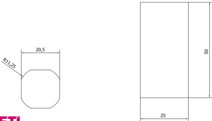
Door drilling
